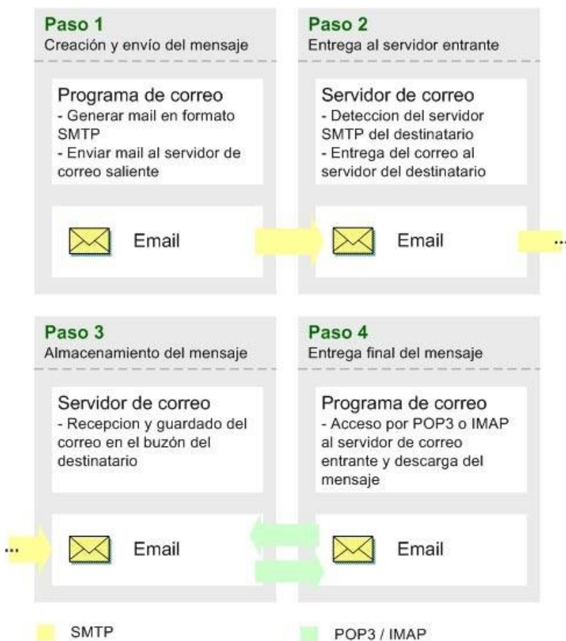
Figura 1. Organización de smtp
