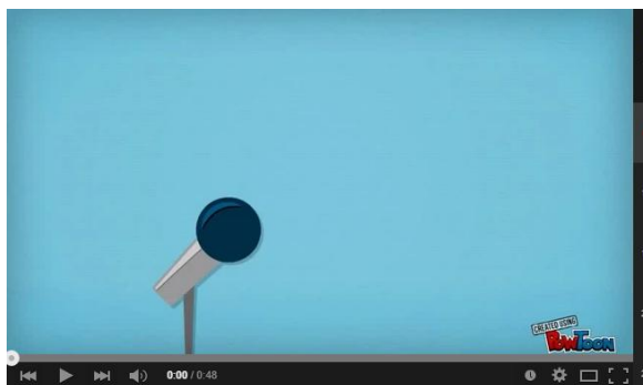
Reacción del Ácido Nítrico con Cobre
