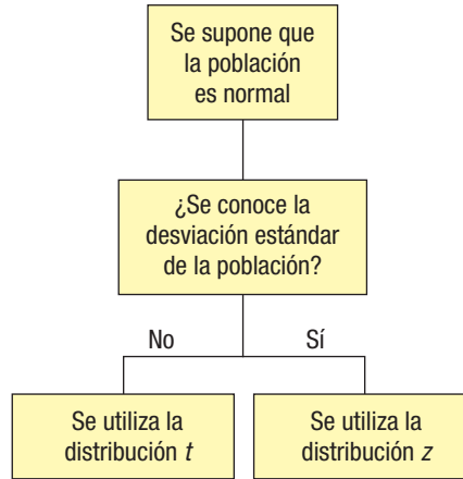
GRÁFICA 9.3 Determinar cuándo usar la distribución z o la distribución t
