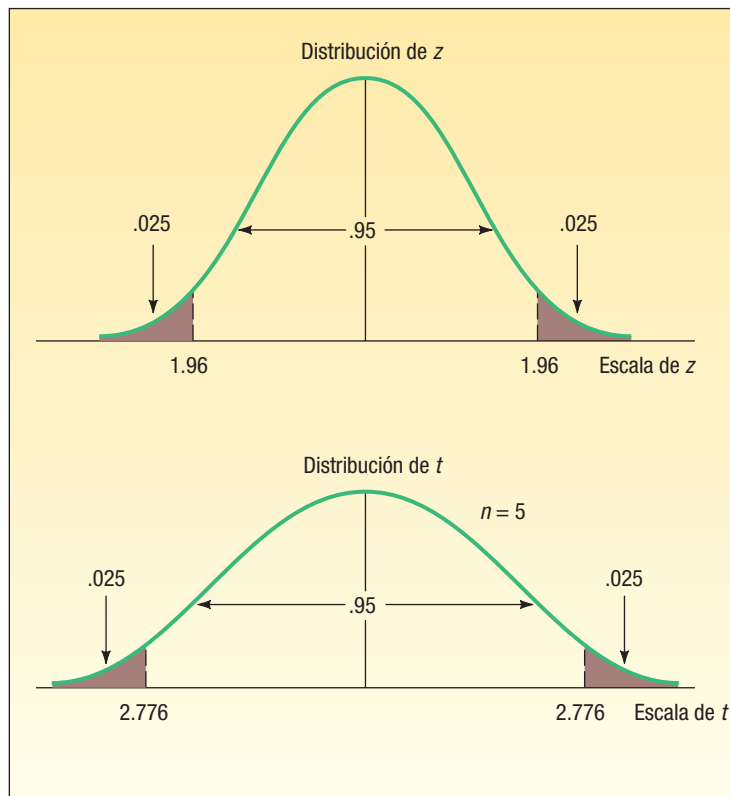
GRÁFICA 9.2 Valores de z y t para el nivel de confianza de 95%
